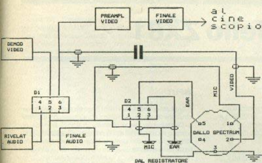
fig. 2: il circuito da realizzare.
